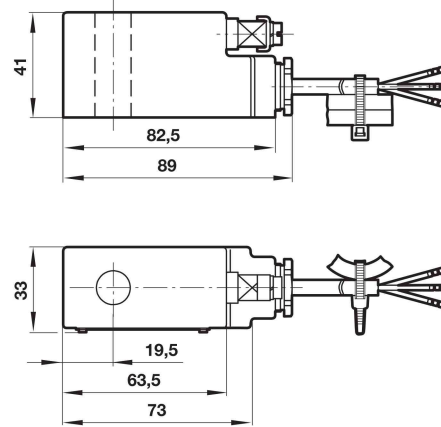
7 Weight: 0,8 kg
