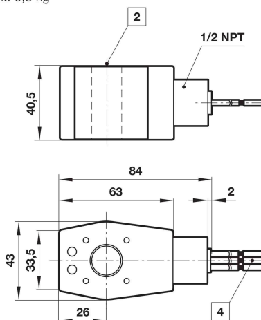
8 Weight: 0,5 kg
