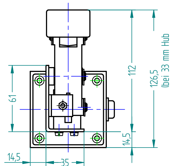
Ansicht X
